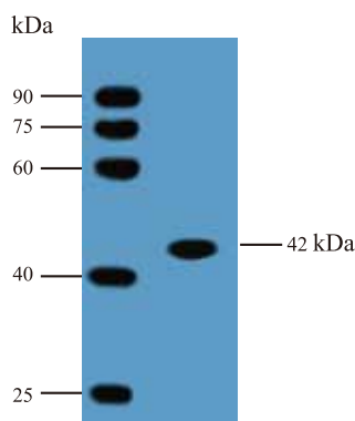
WB: 抗 \beta -Actin鼠单克隆抗体 检测 \beta -Actin蛋白(42 kDa)。
