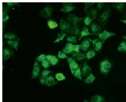
IF: 抗 \beta -Actin鼠单克隆抗体检测HeLa细胞中 \beta -Actin 蛋白的表达。
